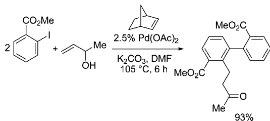
SCHEME 7. 3,2'-Dimethoxycarbonyl-2-(3-oxobutyl)-1,1'-biphenyl
